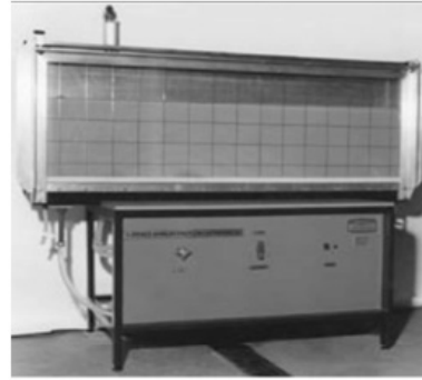
خزان تربة / ماء Soil / Water Model Tank يستخدم لتمثيل الجريان داخل الوسط الترابي كحركة المياه الجوفية ومياه الامطار الساقطة على التربة ... الخ
