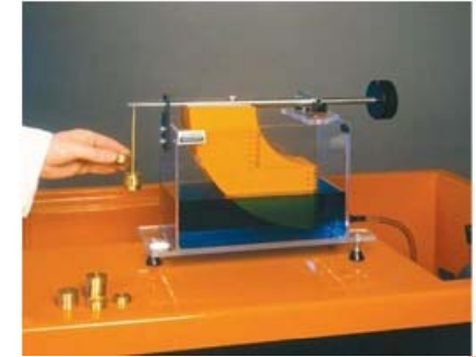
جهاز تمثيل الضغط الهيدروليكي Hydrostatic Pressure Apparatus يستخدم لتمثيل الضغوط والقوى الساكنة على الاجسام المغمورة
